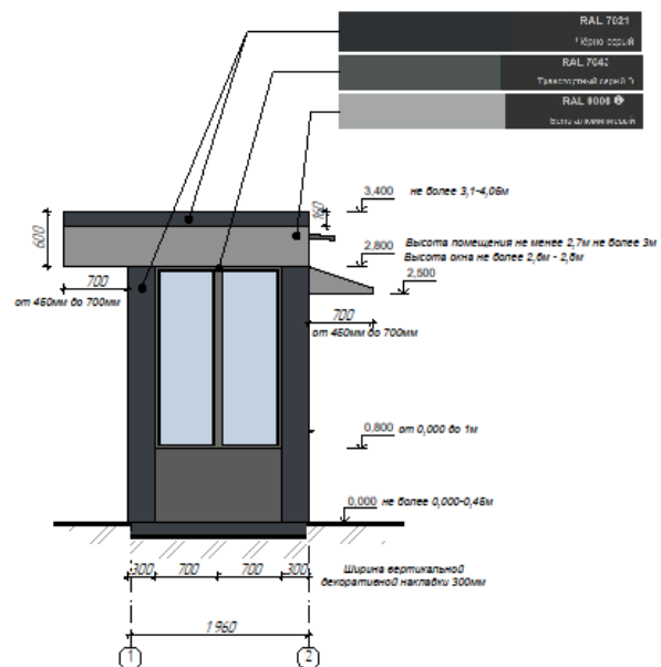
Фасад малого киоска в осях "1-2".
